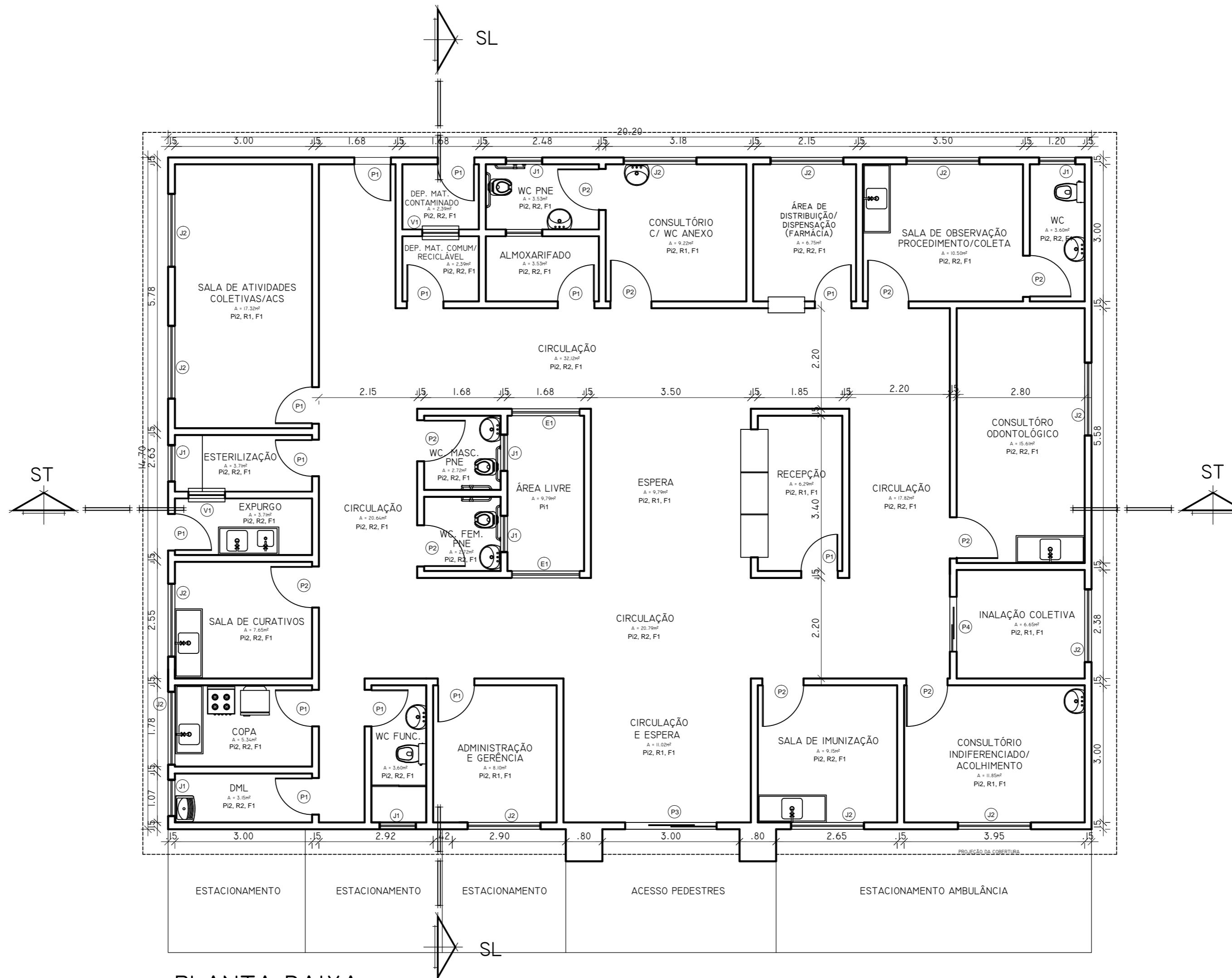
PLANTA BAIXA ESC.: 1/75
