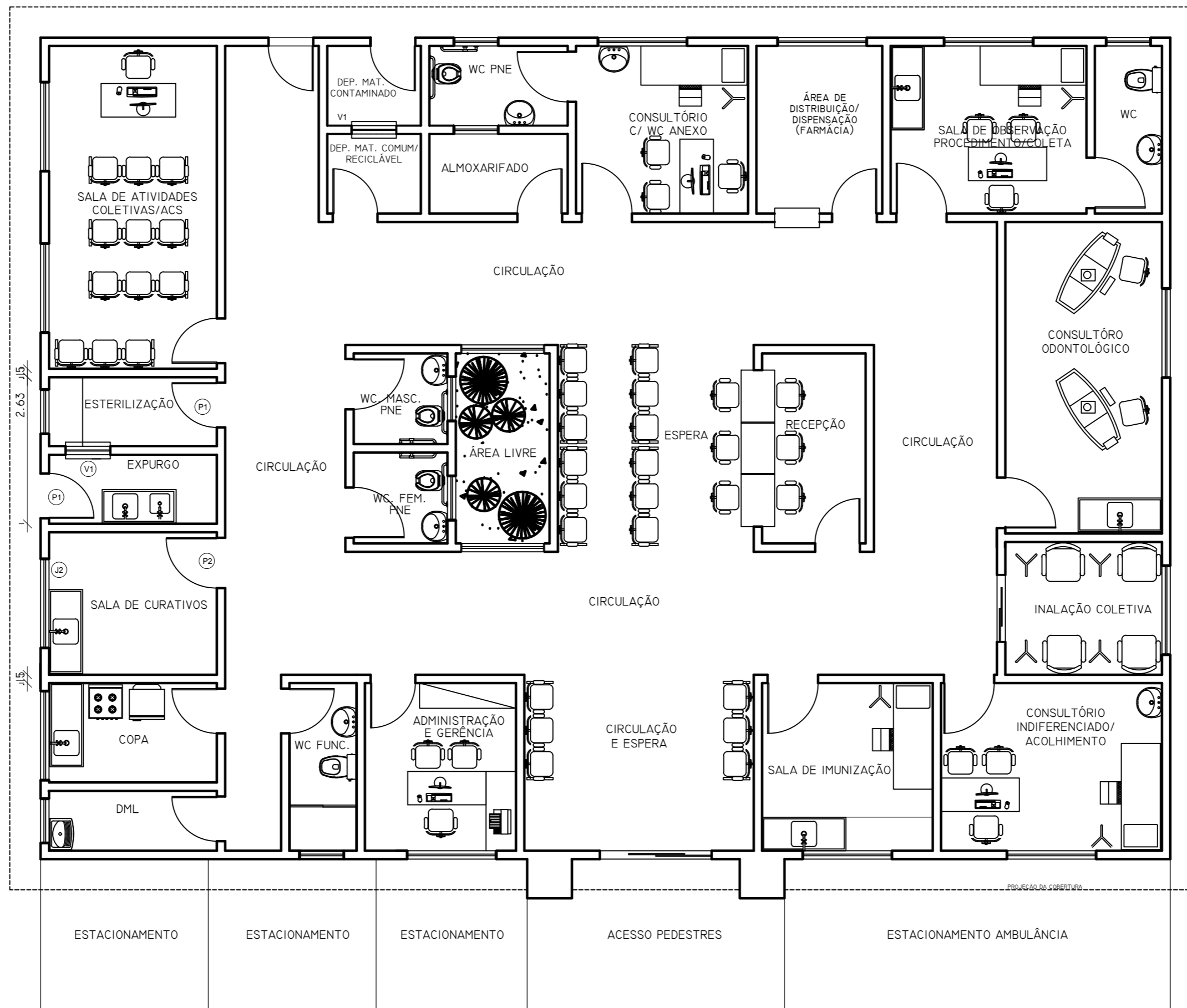
PLANTA BAIXA / LAYOUT ESC.: 1/75
