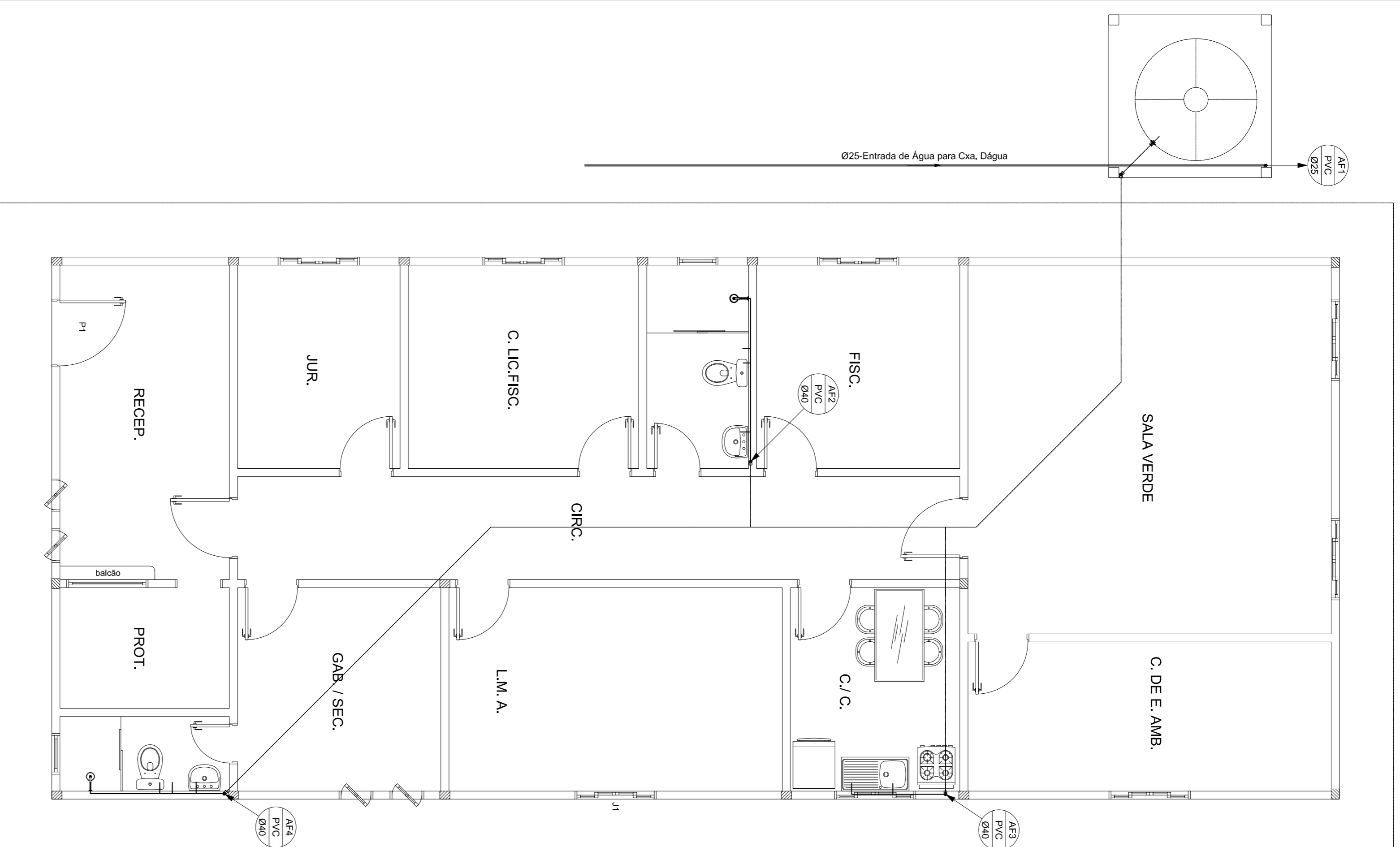
PLANTA BAIXA - HIDRÁULICA
